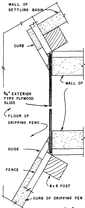
DETAIL "Z" SCALE: 1/2" = 1'-0"
