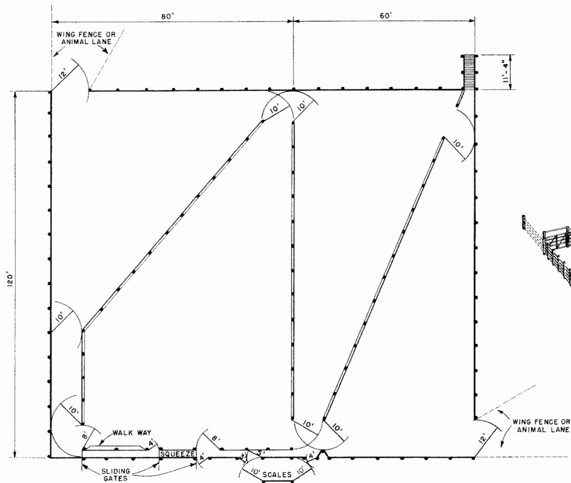
PLAN SCALE: 1/16" = 1'-0"
